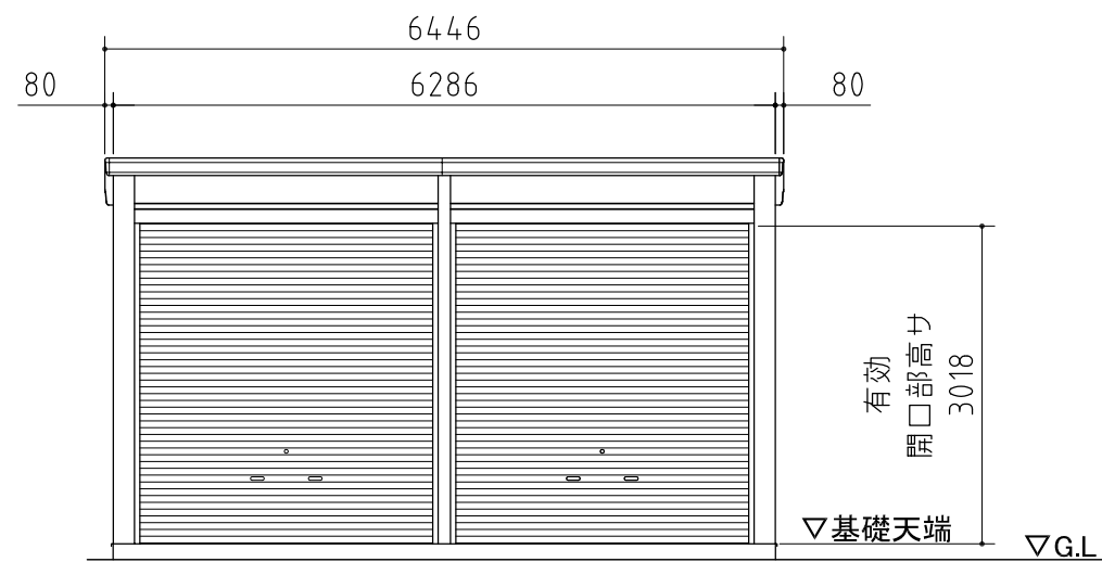
正面図
